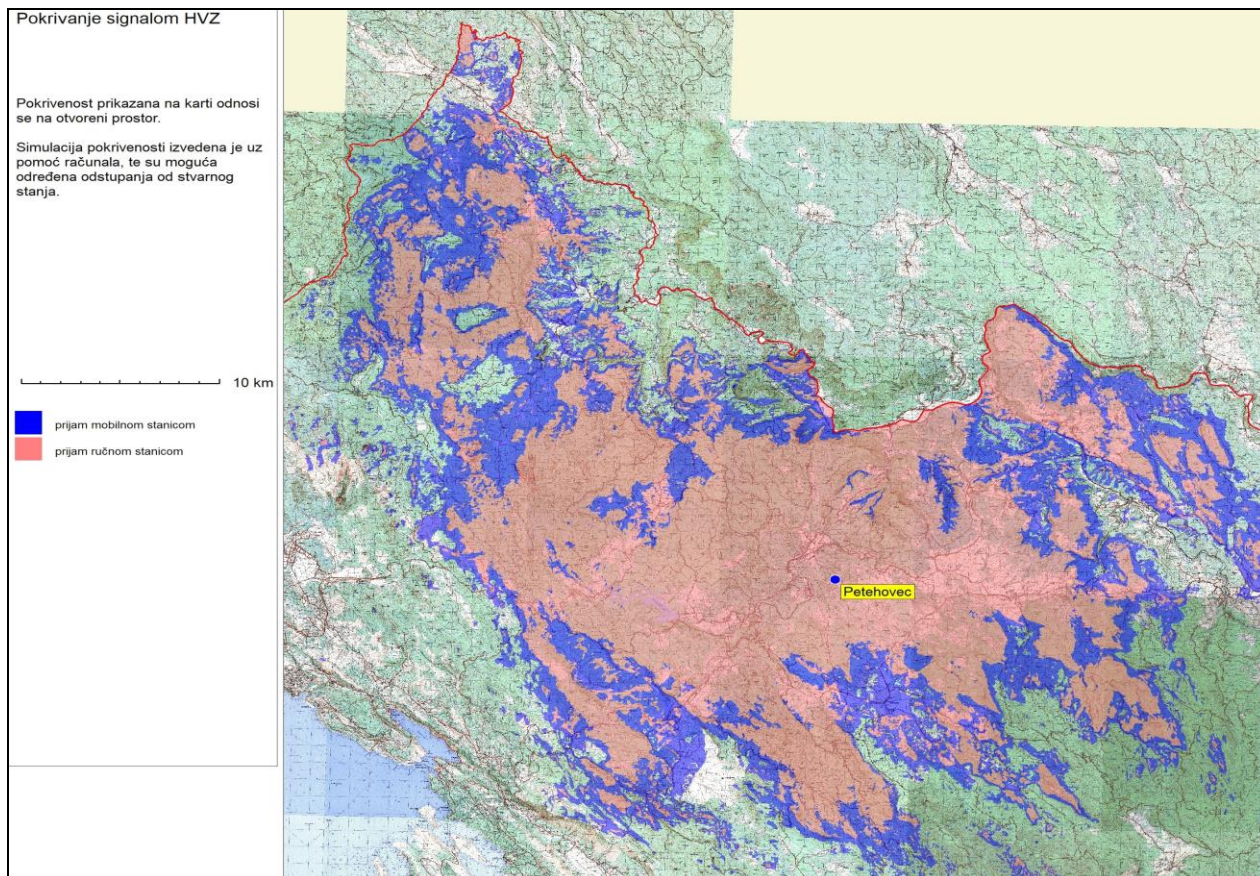
Slika 4. Prikaz pokrivenosti signalom repetitora Petehovac
