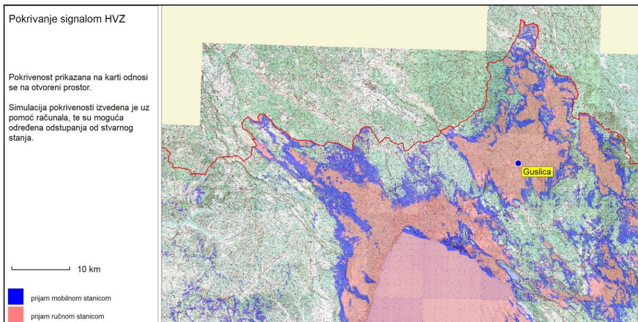
Slika 5. Prikaz pokrivenosti signalom repetitora Guslica
